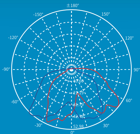
子午面配光曲线
